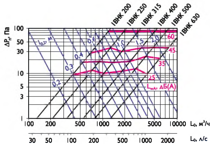
Аэродинамические и акустические характеристики 1ВНК при подаче воздуха в помещении
