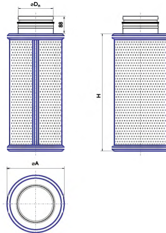
Конструктивная схема воздухораспределителя 1ВНК
