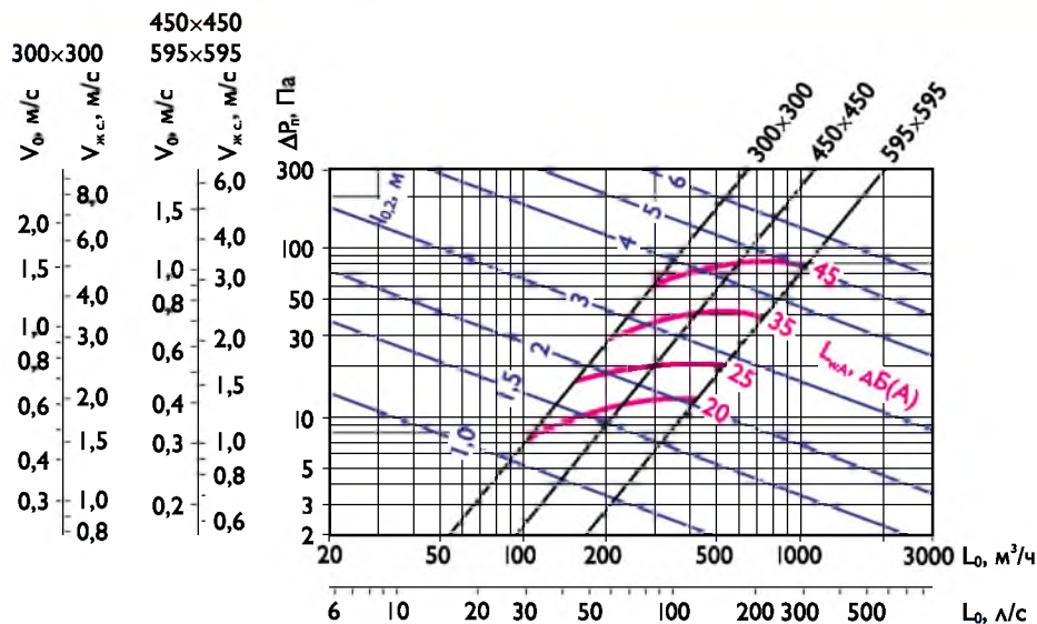
Аэродинамические и акустические характеристики 1СПП, 1СПП-М при подаче воздуха в помещение
