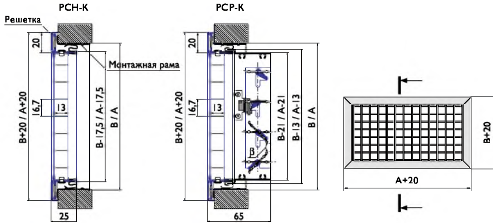
Характеристики решеток РСН-К, РСР-К
