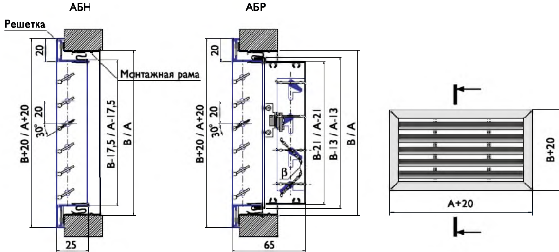
Характеристики решеток АБН, АБР
