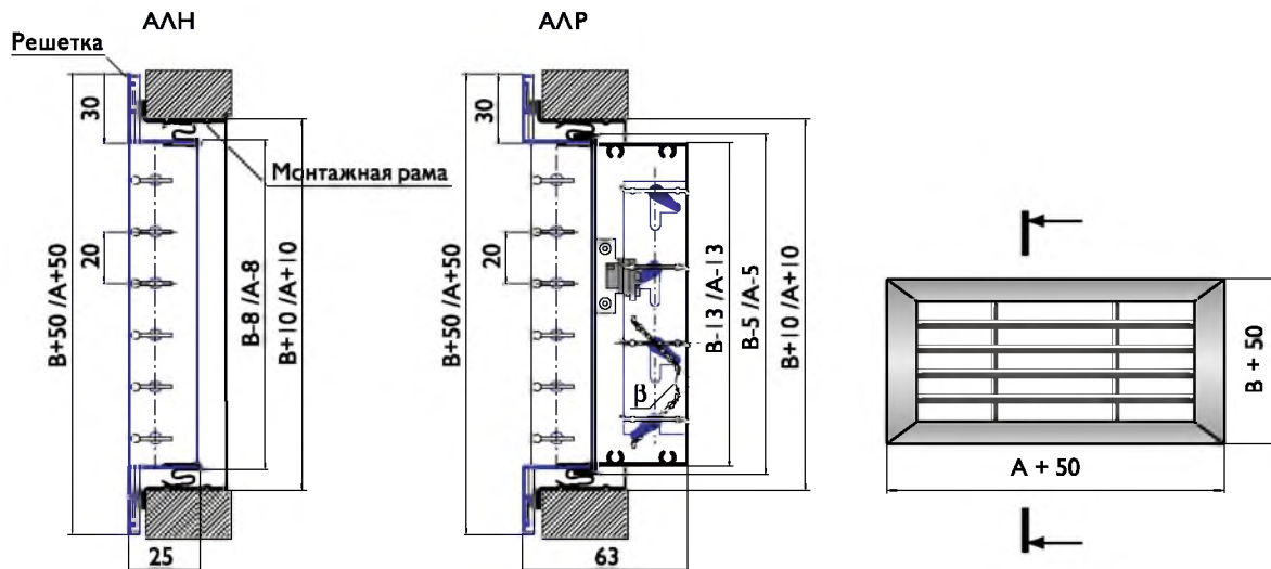
Характеристики решеток АЛН, АЛР
