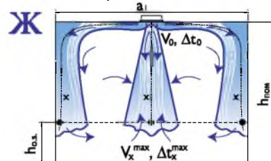
Ж сверху вниз комбинированными струями
