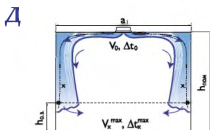
Д сверху вниз настилающимися на потолок веерными струями
