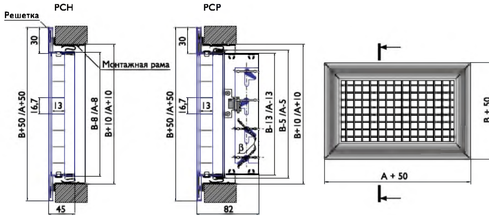
Характеристики решеток РСН, РСР
