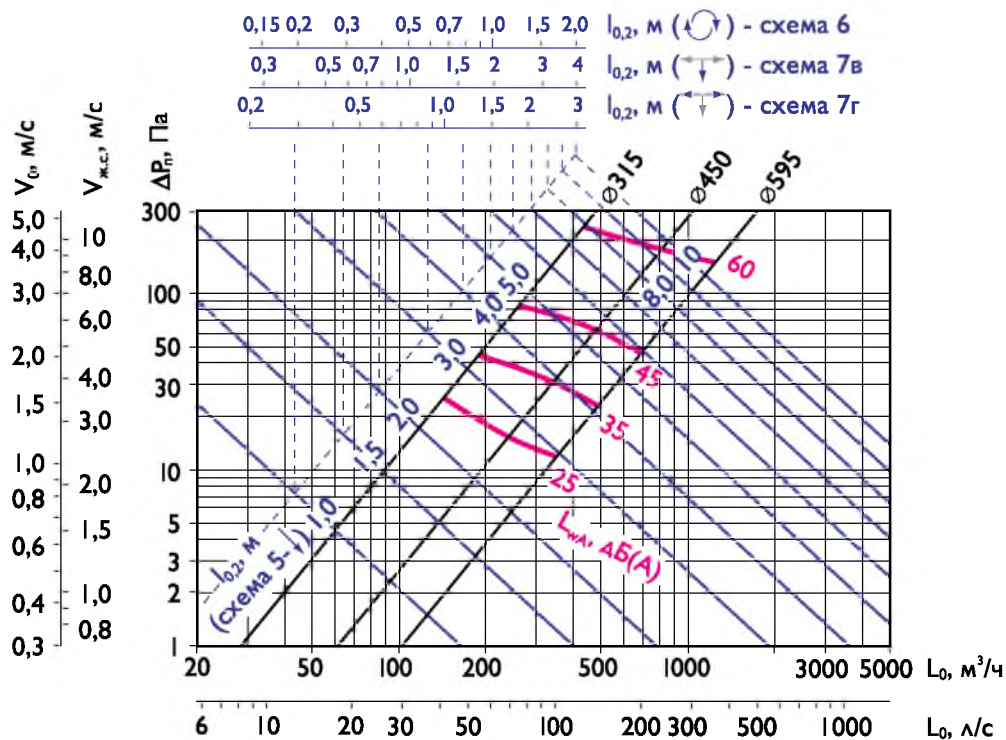
Аэродинамические и акустические характеристики 1BKT при подаче воздуха в помещении коническими, закрученными, комбинированными потоками
